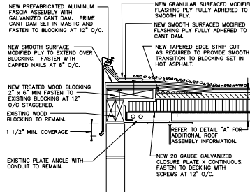
02 ROOF EDGE DETAIL SCALE: 1 1/2" = 1'-0"
